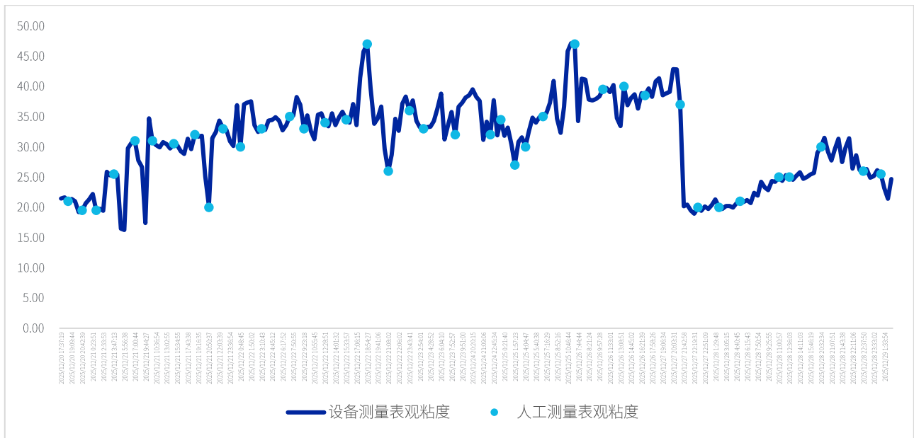
REALology 全自动旋转粘度计的表观粘度 (AV) 与标准现场流变仪 (范氏 35 型) 的读数对比
