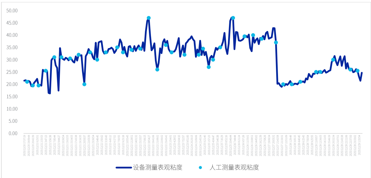
REALoogyFAST 的表观粘度 (AV) 与标准现场流变仪 (范氏 35 型) 的读数对比
